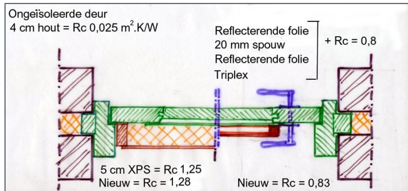
Figuur 8. Omdat het oppervlak van de rest van de deur veel groter is dan de glasruit alleen, verdient het aanbeveling om het slecht isolerende paneel aan de onderzijde ook nog te isoleren.
